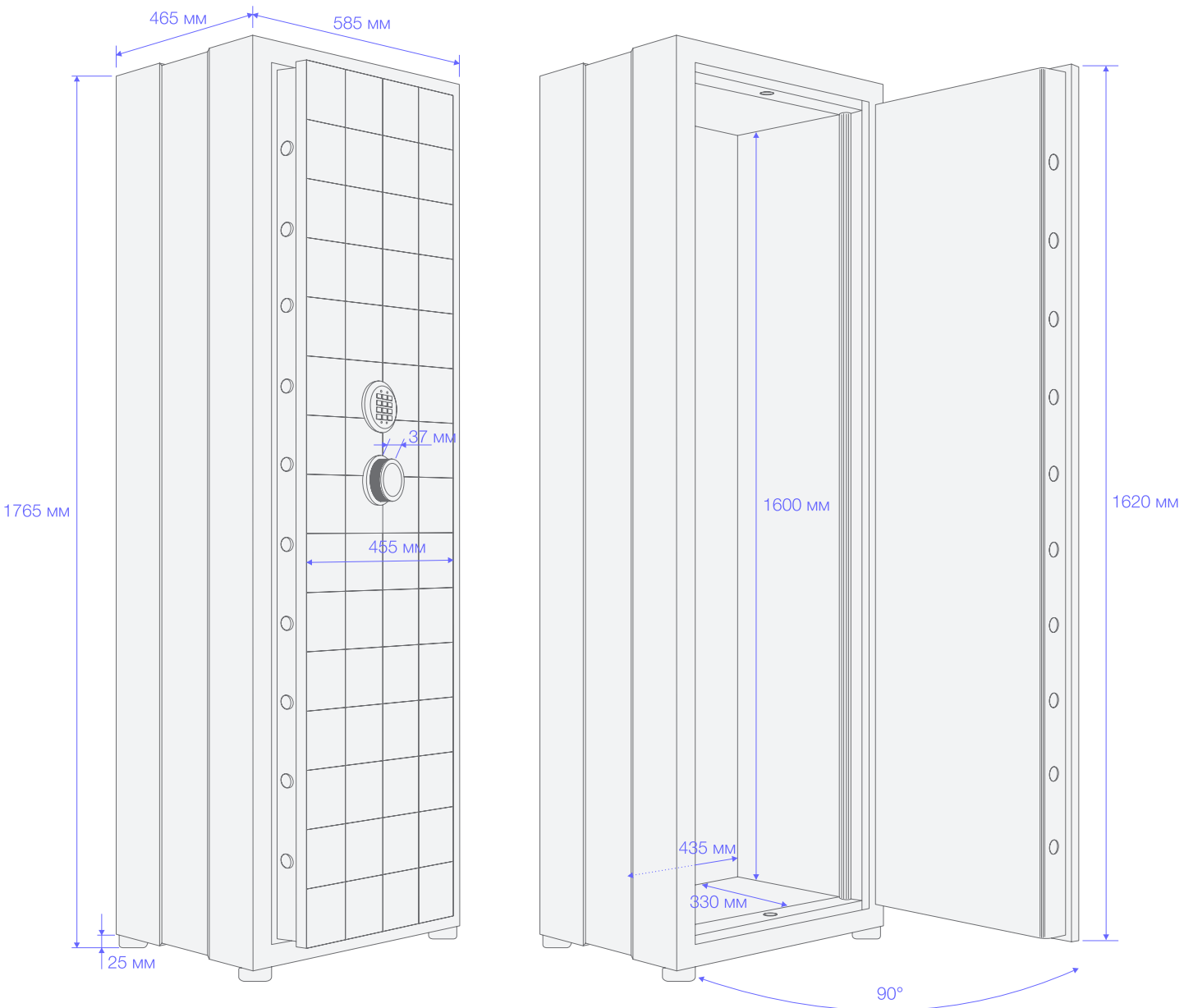
Отдельностоящий сейф AGARTIS SIRIUS I
