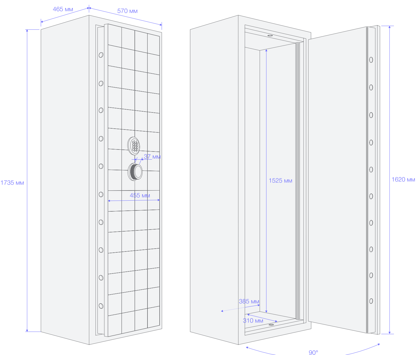
Встраиваемый сейф AGARTIS SIRIUS I
